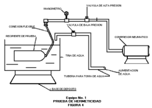
Equipo No. 1 PRUEBA DE HERMETICIDAD FIGURA 4
